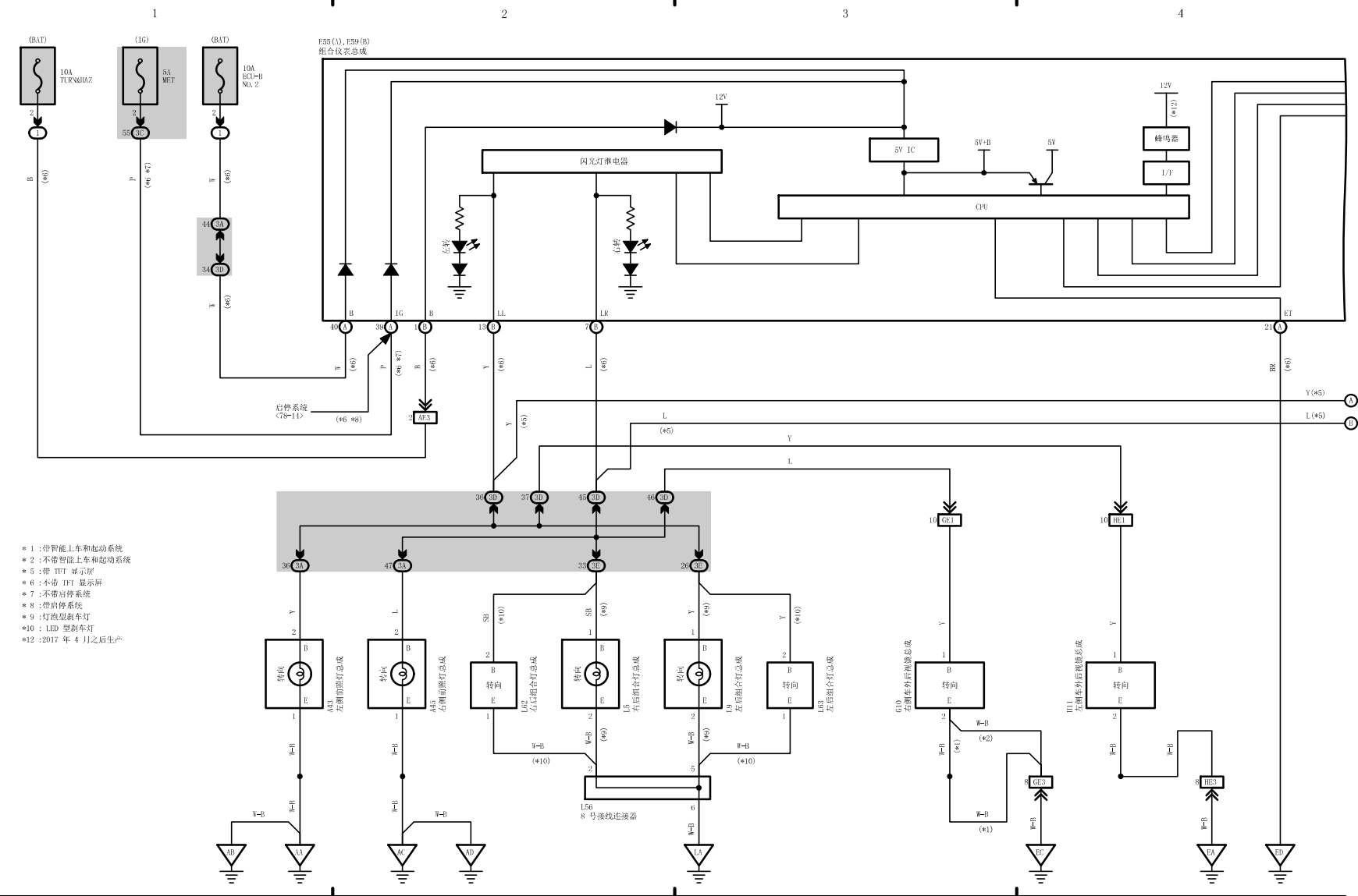
转向信号和危险警告灯 (GTMC 制造)
